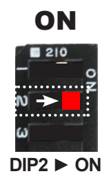
ES - Configuración del tipo de carga
