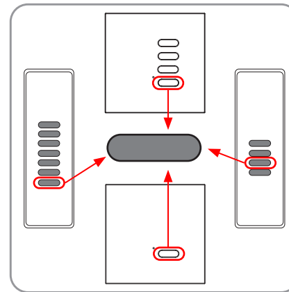
ES - Canal simple de mando: función ON, OFF o ON/OFF/DIM
